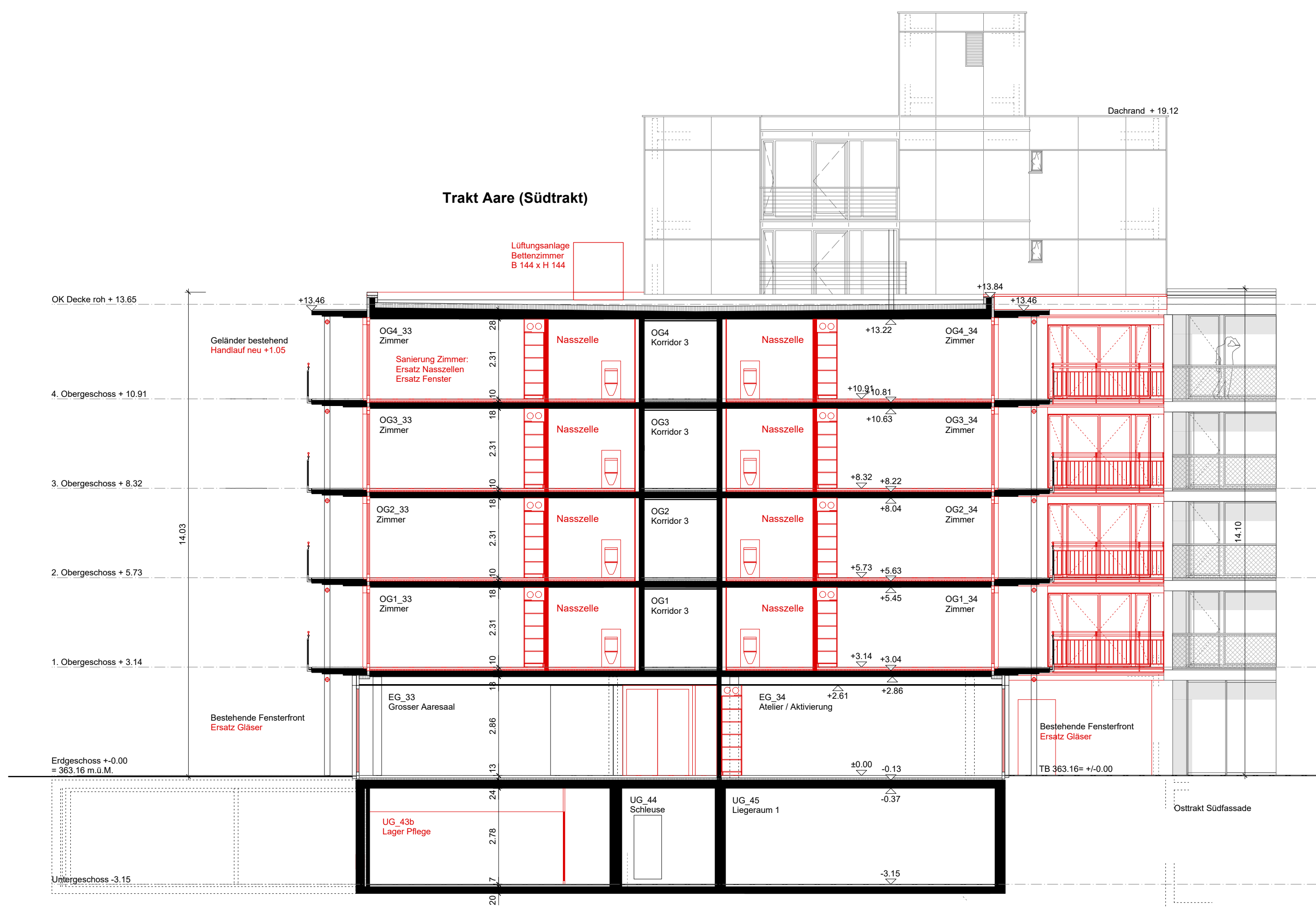
Gesamtanlage Querschnitt L-L
