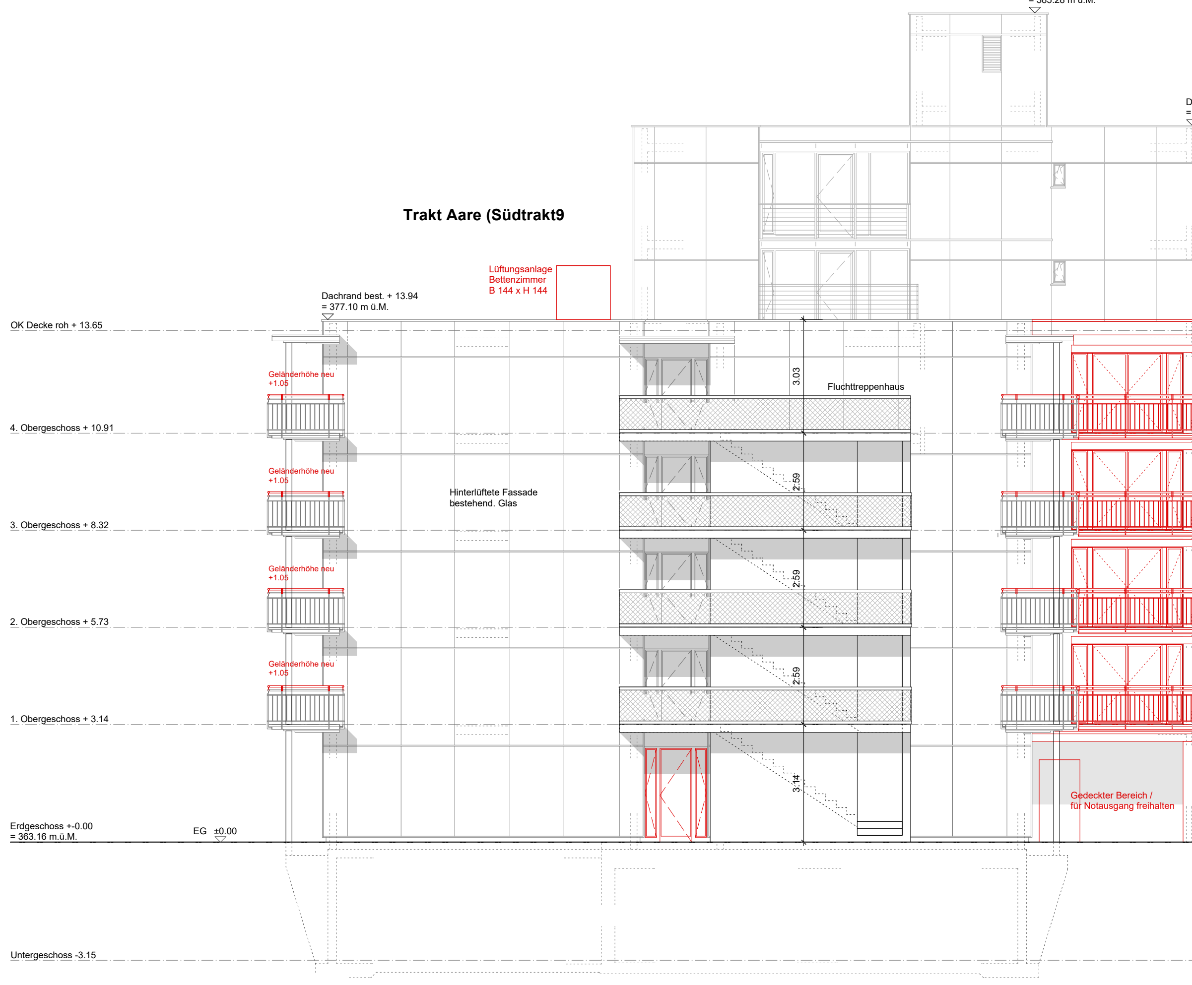
Gesamtanlage Südfassade
