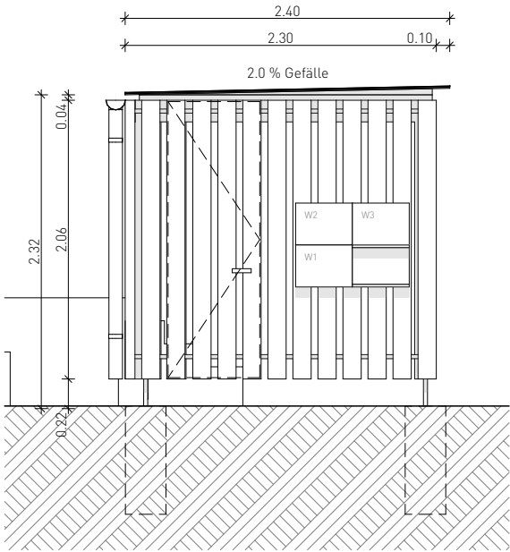
Westansicht
