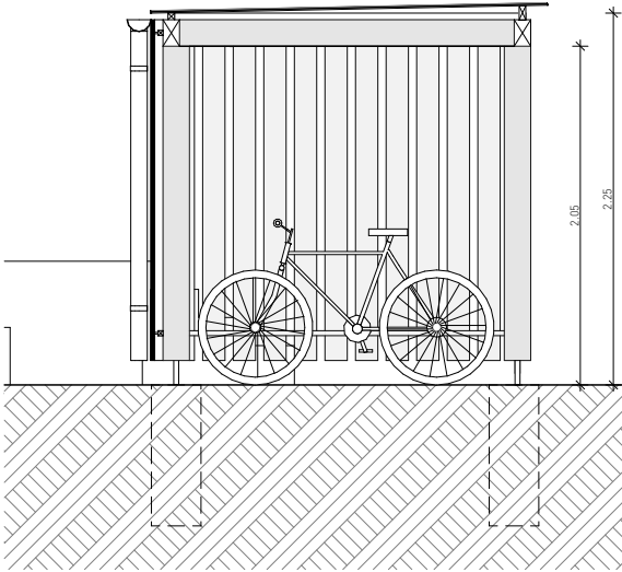
Querschnitt
