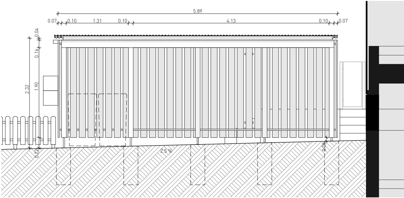
Südansicht
