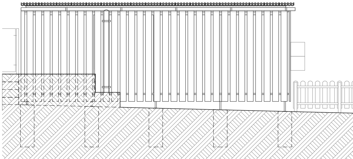
Nordansicht
