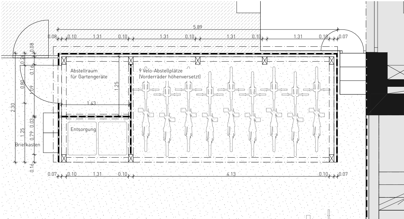
Grundriss
