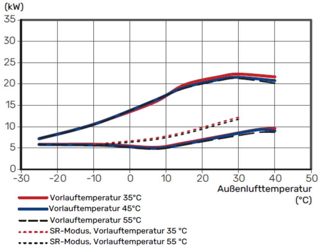
S2125-16 max. und min. Heizleistung in kW
