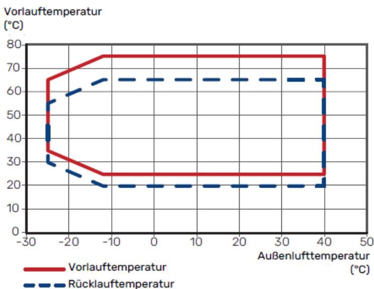
S2125-16 Betriebsbereich Heizung
