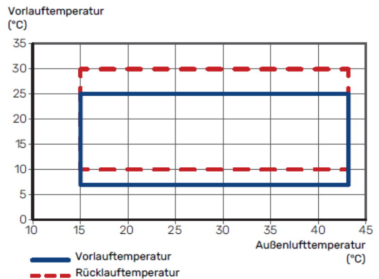
S2125-16 Betriebsbereich Kühlung
