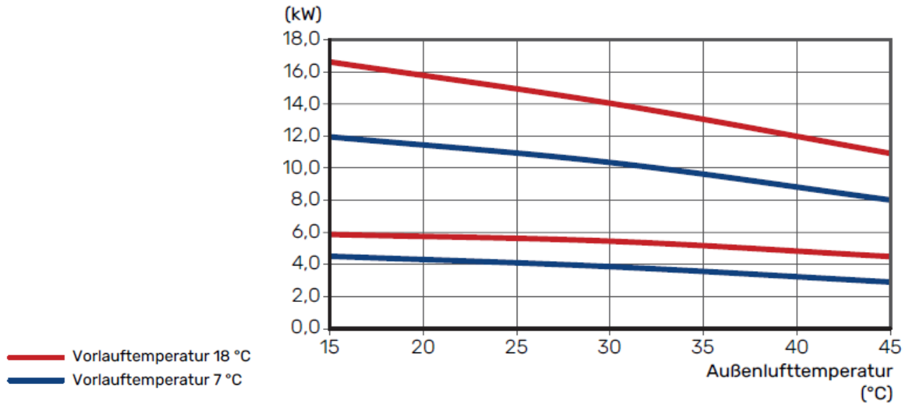
S2125-16 max. und min. Kühlleistung in kW
